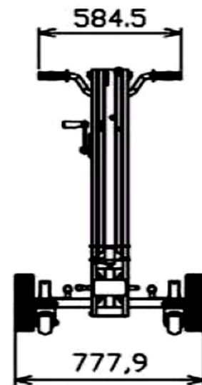
Roues à empattement réglable
